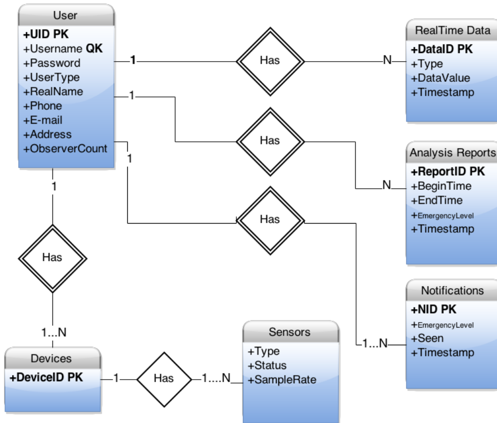
Figure 9 ER Diagram
